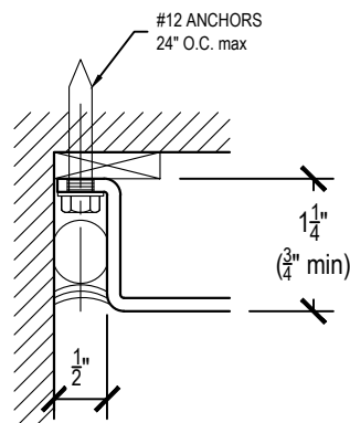
JAMB DETAIL
