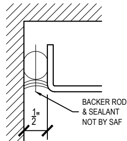
JAMB DETAIL
